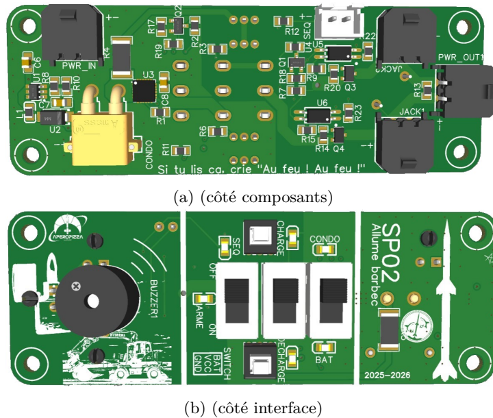
FIGURE 1.3 – Rendu 3D de la carte allumage principale
